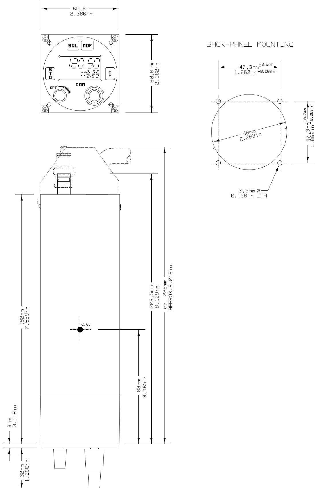
Abb. 2-3 Einbaumaße VHF-Sprechfunkgerät
